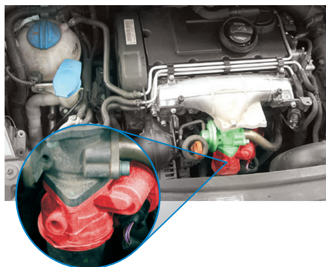
Вид моторного отсека VW Touran выделено зеленым: клапан EGR; выделено красным: регулирующая заслонка
